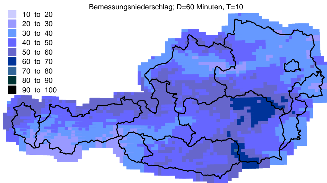
Abbildung 6: Bemessungsniederschläge [mm] für die Dauerstufe 60min und die Jährlichkeit 10
